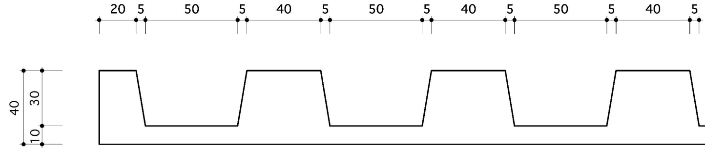
断面拡大図 S=1/2
